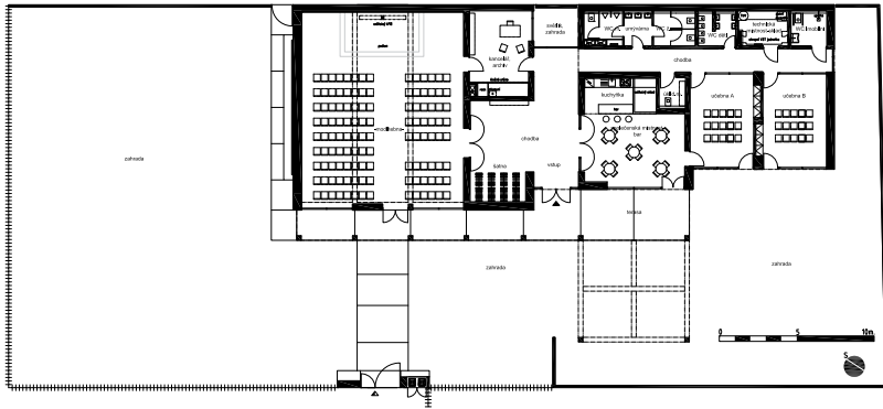
PŮDORYS
